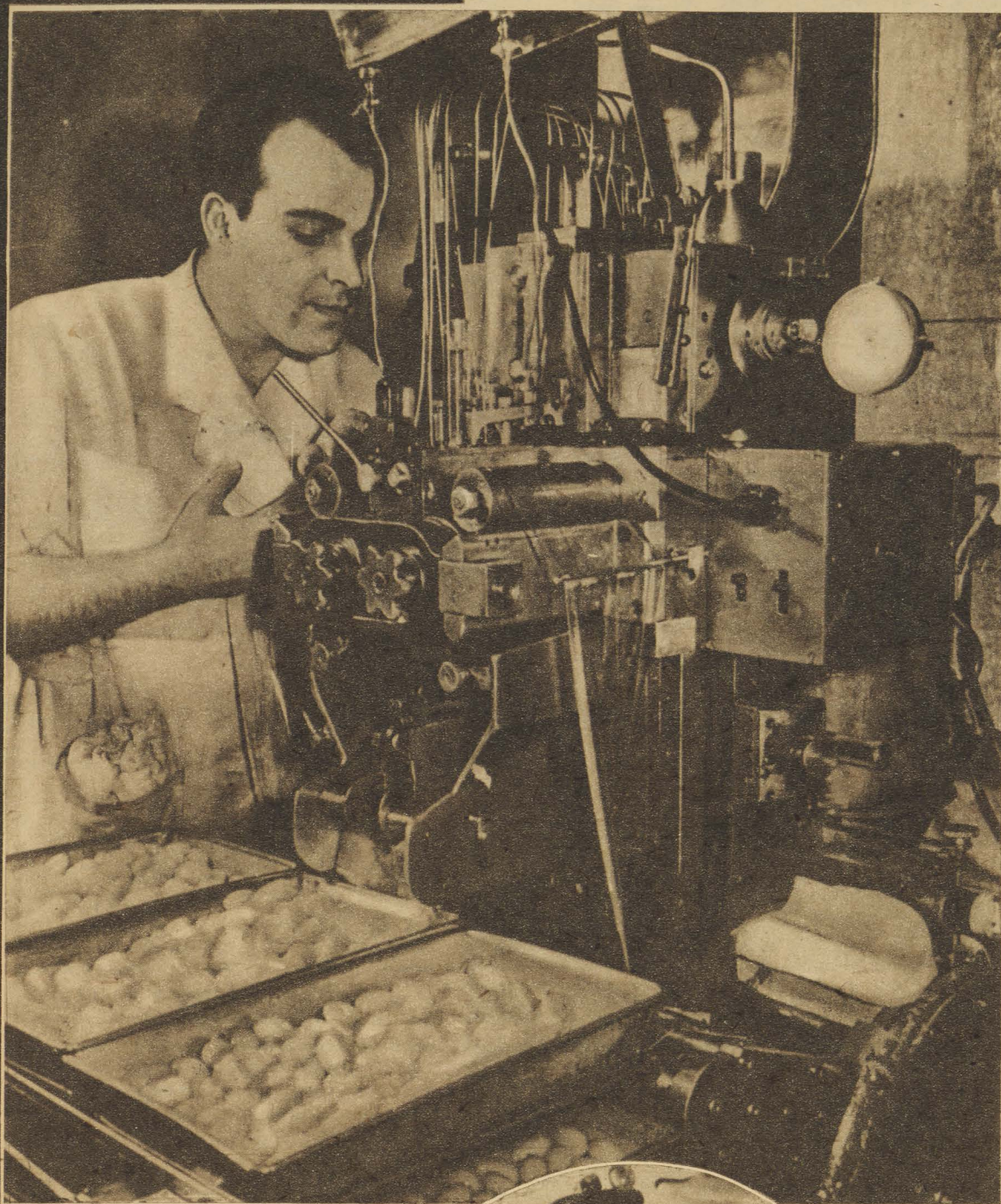
Ἀπὸ τὴν μηχανὴν αὐτὴν ἡ ζελατίνη ἐξέρχεται χρωματισμένη καὶ συγχρόνως τὰ διάφορα βιταμινοῦχα καταπότια λαμβάνουν ὀρισμένα σχήματα.
