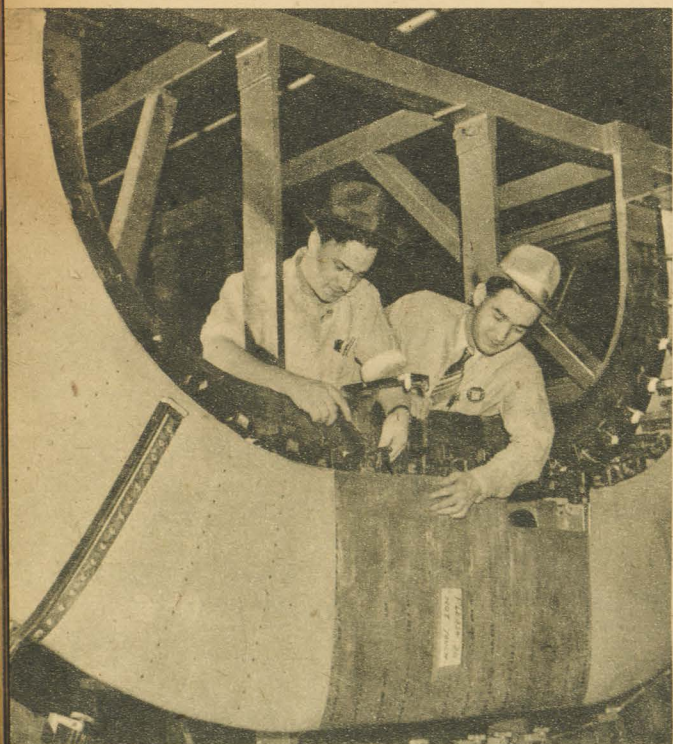
Ἡ ἀποπεράτωσις ἐνὸς βομβαρδιστικοῦ εἰς τὸ νέον ἐργοστάσιον τοῦ Χένρυ Φόρντ εἰς Οὐίλλω Ράν.
