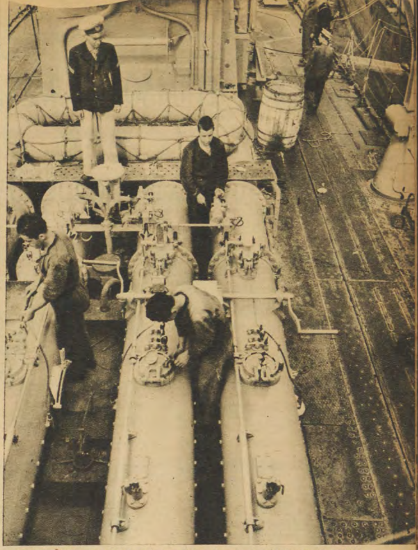
ΜΕΤΑ ΤΗΝ ΔΡΑΣΙΝ: Οἱ τορπιλλοβλητικοὶ σωλήνες τῆς «Βασίλισσας Ὀλγας» καθαρίζονται ἀφοῦ ἔδωκαν ἓνα σκληρὸ μάθημα εἰς τὸν ἐχθρόν.
